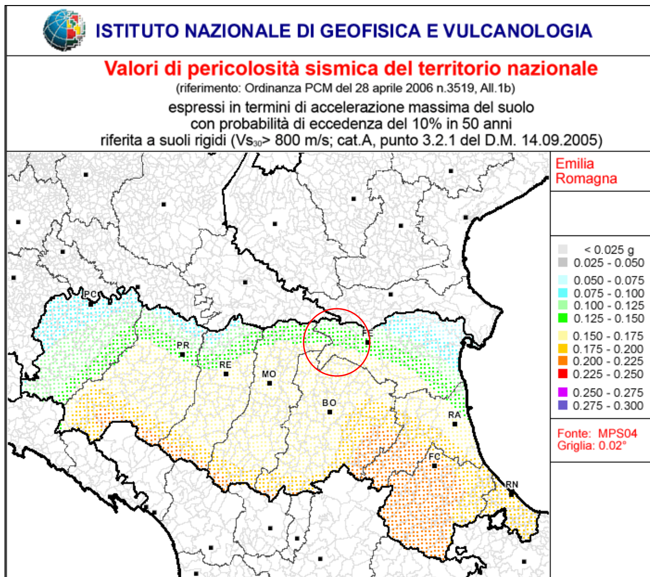
Figura 1.3.1.1-1 Zonizzazione sismica Emilia-Romagna
